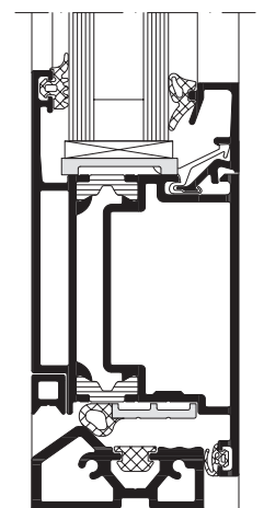
Porta Schüco ADS 50, scala 1:2 Schüco Door ADS 50, scale 1:2
